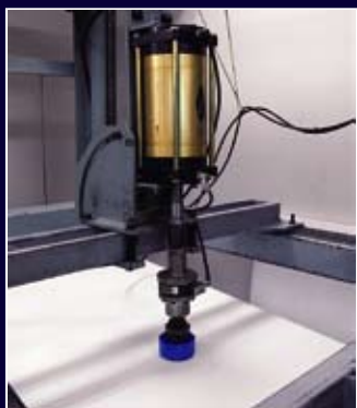
試験風景 (写真は集中荷重試験)
