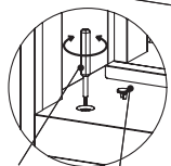
プラスドライバー 樹脂製キャップ
